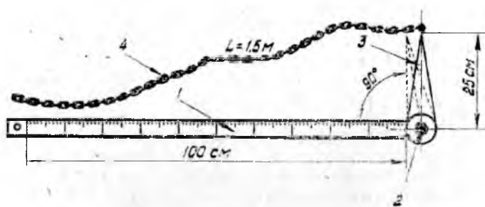
Рис. 2. Ледомер
