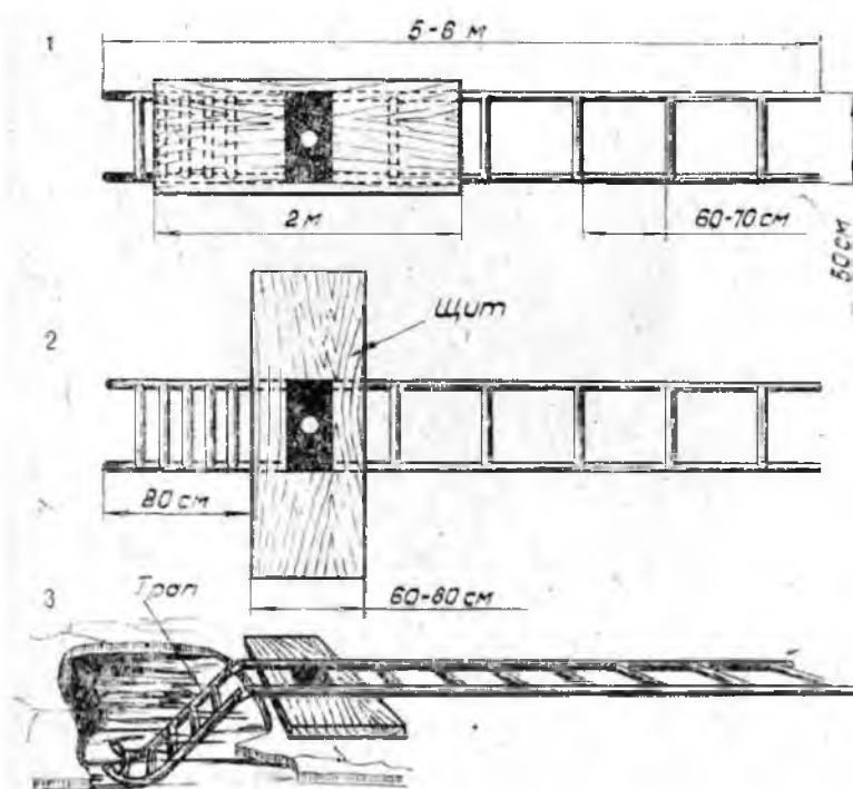
Рис. 10. Спасательная лестница № 2.
